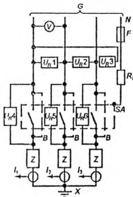
Схема испытательной цепи для проверки включающей и отключающей способности трехполюсного аппарата
