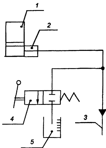
1 – гидроцилиндр подъема стрелы; 2 – специальное регулирующее устройство на случай разрыва гидролинии; 3 – гидрораспределитель; 4 – устройство, имитирующее отказ; 5 – мерный сосуд.
