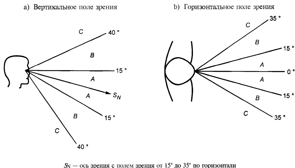
Рисунок 2 — Задача наблюдения сигнала
