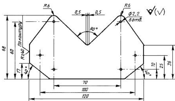
Рисунок 5 - Развертка угольника
