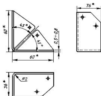
Рисунок 4 - Угольник
