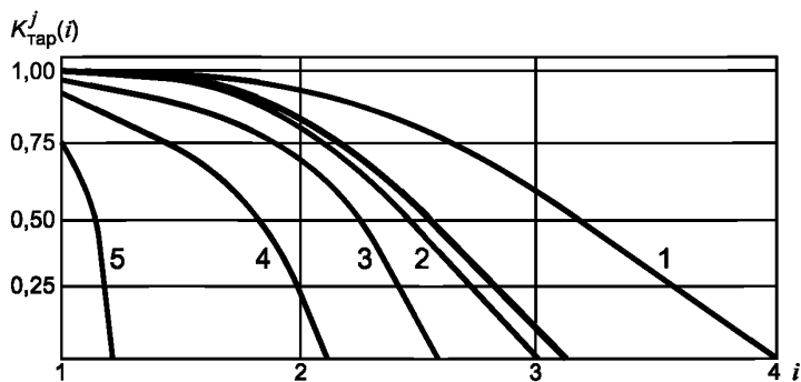
Рисунок 2 — Зависимость K^j(i) , нанесенная на серию тарифовочных кривых
